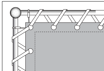
Verspannung des Druckes an einem vormontierten Rahmengestänge
