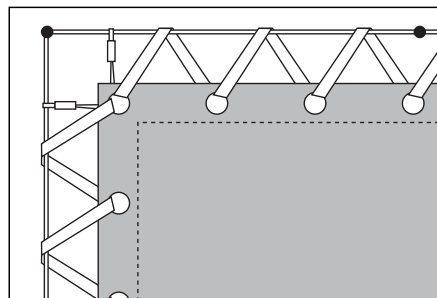
Verspannung des Druckes an einem vormontiertem Drahtseil
