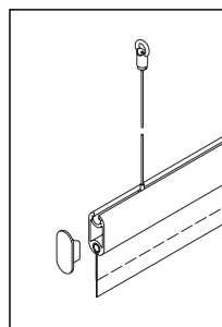
Abhängung mit Seilhalter und Öse, höhenverstellbar
