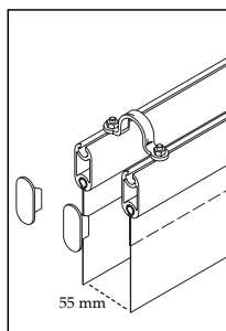
Verbindungsstück für Doppelbanner
