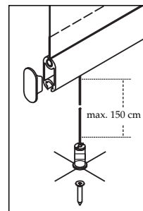
Bodenanker mit verstellbarer Seilklemme
