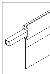
Verbindung mit Schäftungskern, 15x15 mm
