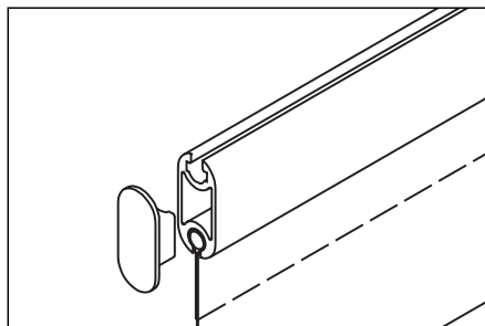
Kederprofil KP46 mit Abdeckkappe und Kederschlauch
