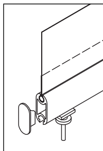
Haltewinkel mit Spannschraube, unten
