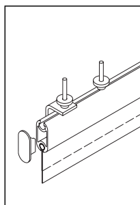
Haltewinkel mit Spannschraube, oben
