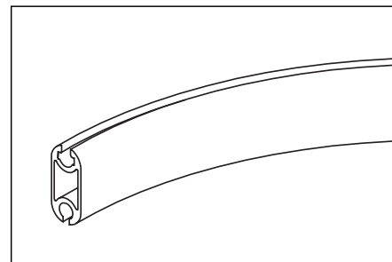
Kederprofil KP46, gebogen
