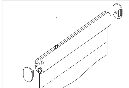
Kederprofil KP28 mit Abdeckklappe mit Kederschlauch
