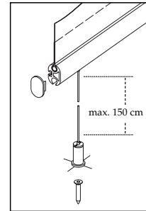
Bodenanker mit verstellbarer Seilklemme
