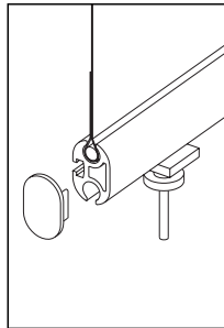
Haltewinkel mit Spannschraube, unten
