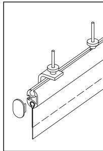
Haltewinkel mit Spannschraube, oben
