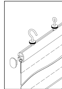
Abhängung mit Haken oder Öse von oben
