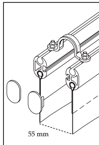
Verbindungsstück für Doppelbanner
