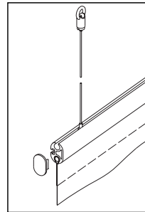
Abhängung mit Seilhalter und Öse, höhenverstellbar
