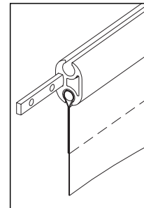
Verbindung mit Schäftungskern, hoch
